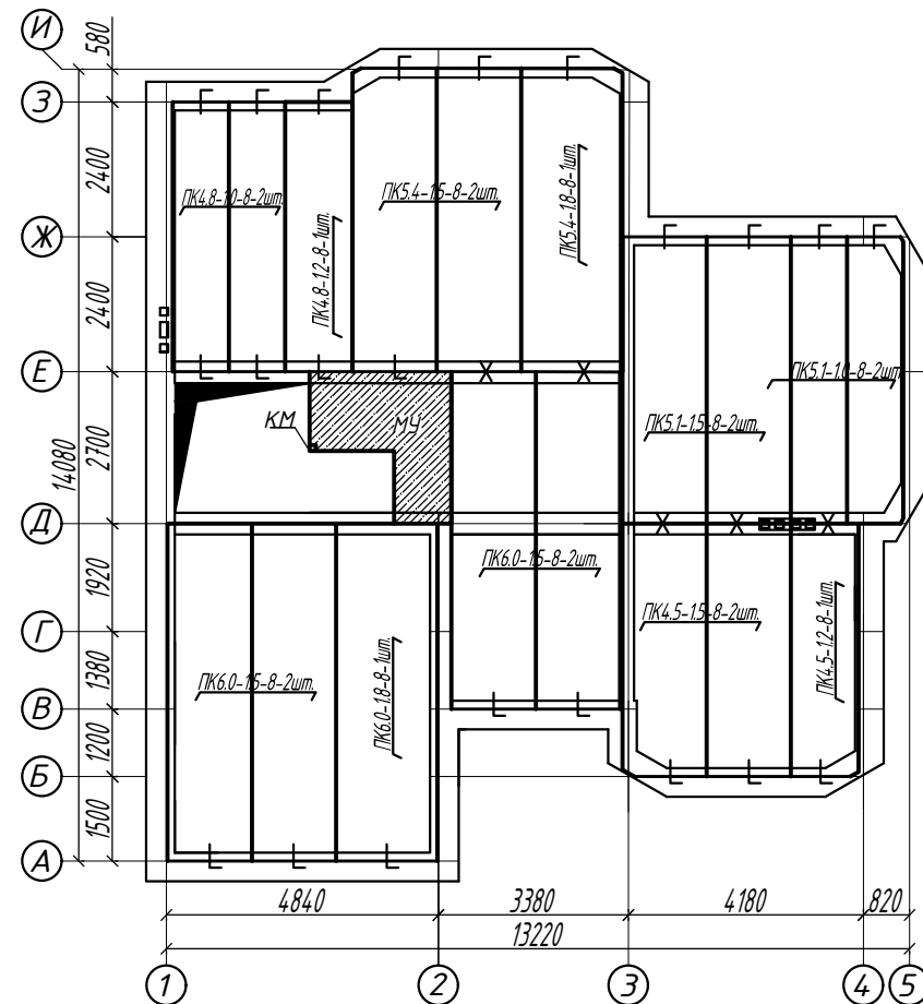
План плит перекрытий на отметке - 0.300
